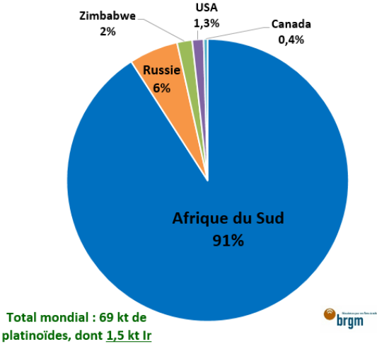
Estimation des réserves de platinoïdes en 2019 (Source : USGS, 2020)
